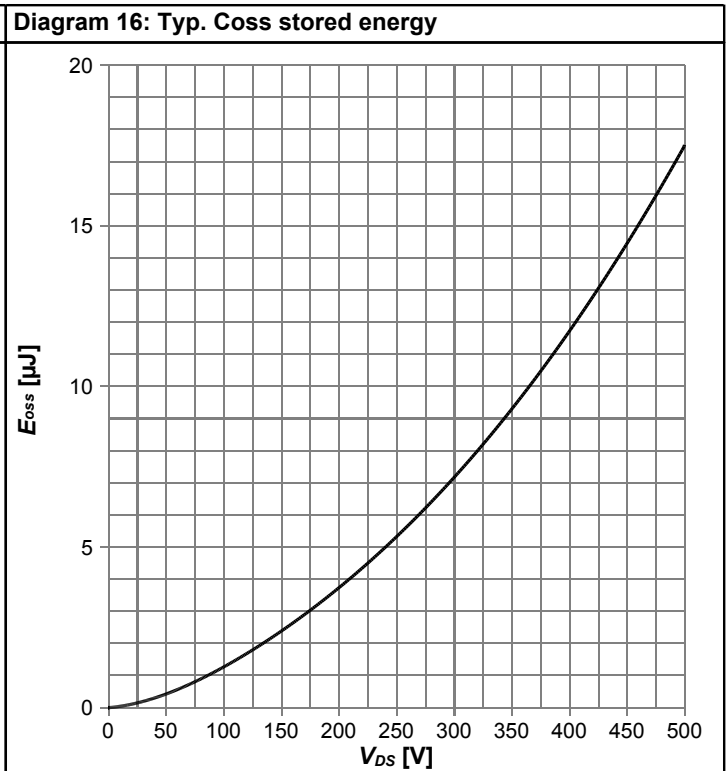
E_{oss}=f(V_{DS})
