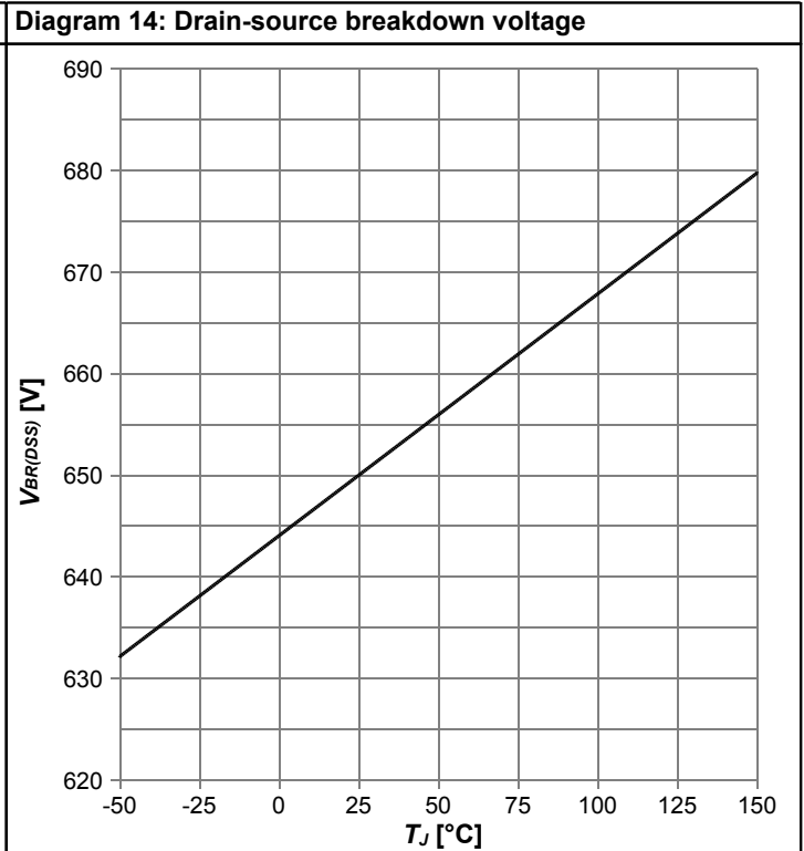
V_{BR(DSS)}=f(T_J) ; I_D=0.6 mA
