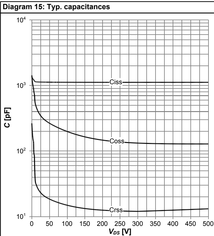
C=f(V_{DS}) ; V_{GS}=0 V; f=250 kHz
