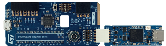
STM32C0316-DK Mini evaluation board
