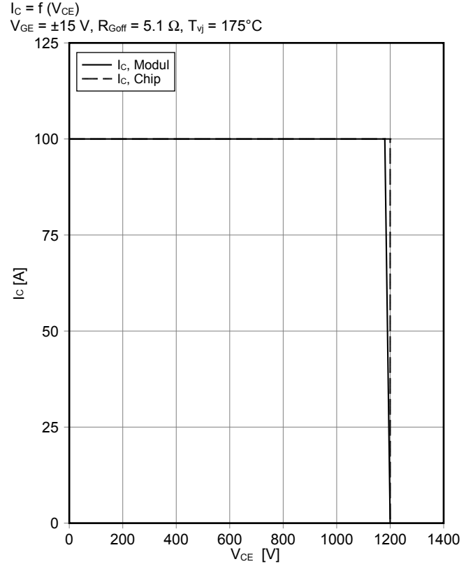
Sicherer Rückwärts-Arbeitsbereich IGBT, Wechselrichter (RBSOA) reverse bias safe operating area IGBT, Inverter (RBSOA) I_C = f(V_{CE})
