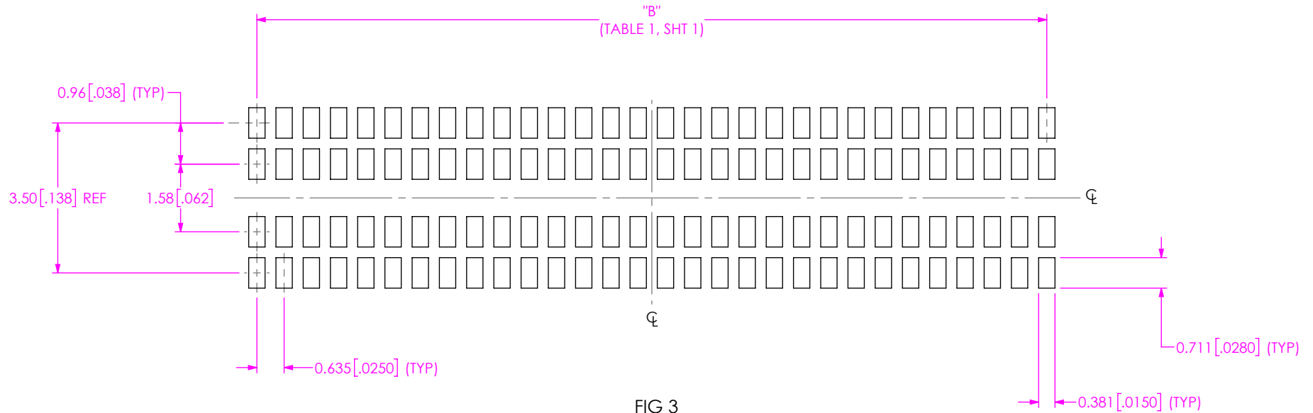
FIG 3 ADF6-30-XX.X-XXX-4-0-A STENCIL SHOWN
